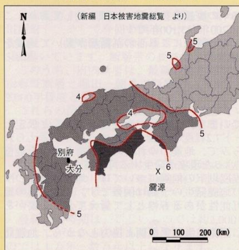
海溝型と活断層型（内陸で発生）の震度分布図（平成16年大分県地域活断層調査研究委員会報告資料）
