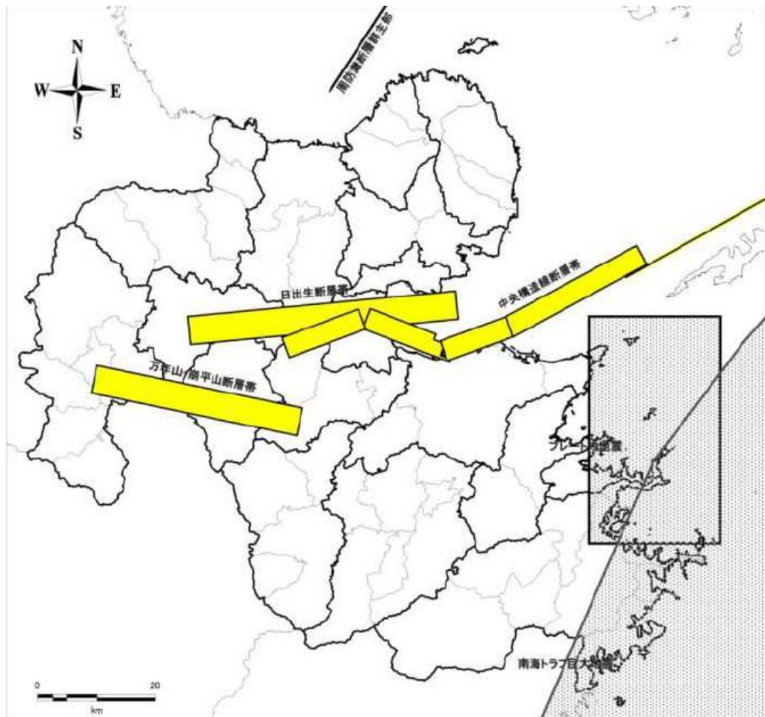
地震位置図
