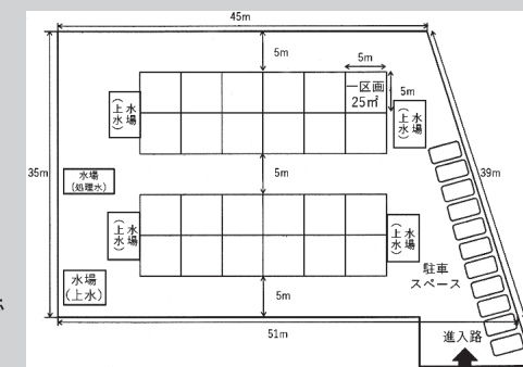
区画図
