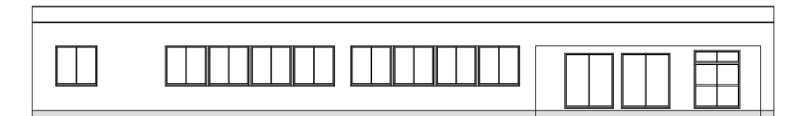
東立面图
