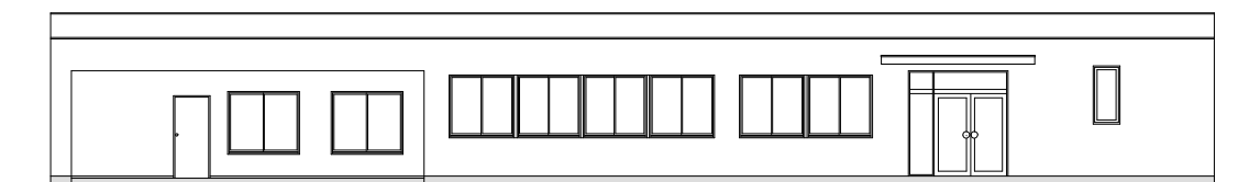
北立面图
